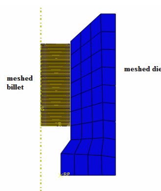
Fig. 3. FEM model
